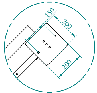
DETTAGLIO A
