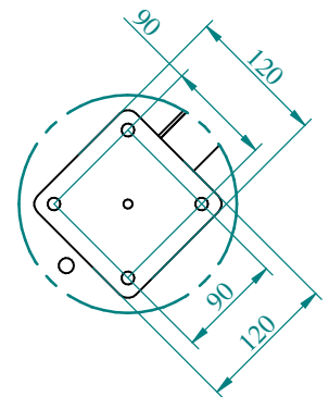
DETTAGLIO B
