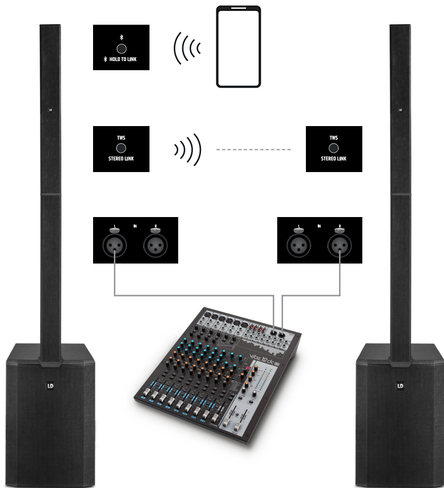
Unidad esclava
